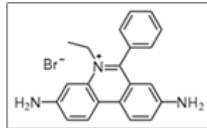
Figure 3.4. Structure chimique du Bromure d'éthidium (BEt)
